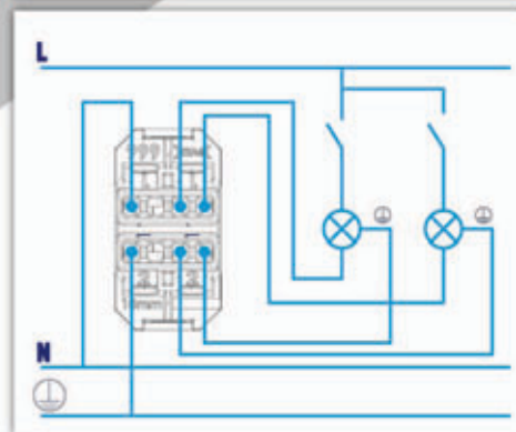
SCHEMA ELETTRICO PUNTO LUCE 3
