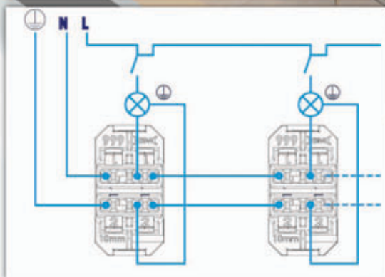
SCHEMA ELETTRICO PUNTI LUCE 1 E 2
